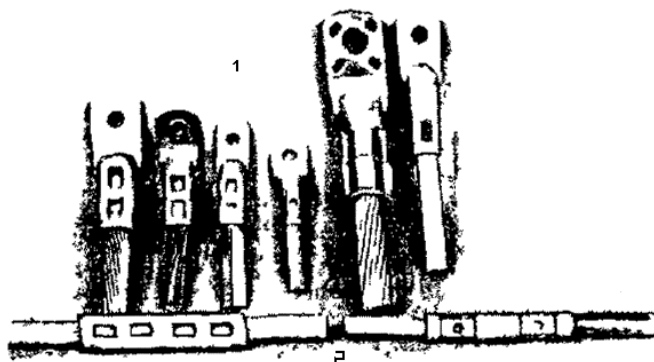
Рис. 27. Образцы оконцевания алюминиевых жил кабелей, выполненные способом опрессовки:
