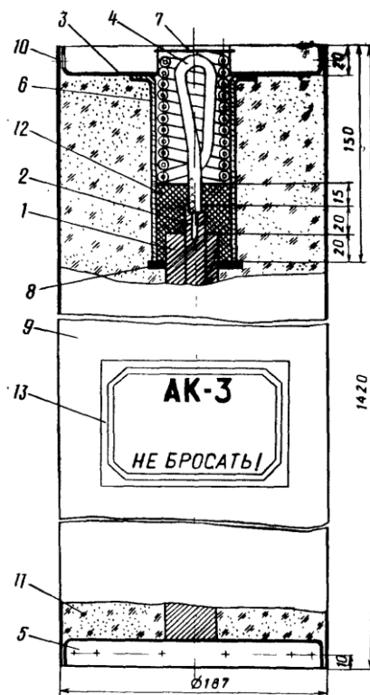
Рис.3. Заземлитель анодный АК-3:
