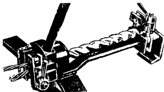
Рис. 4. Приспособление типа МИ-189А для соединения проводов в овальных соединителях методом скрутки
