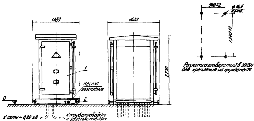
Рис.1. Общий вид смонтированного устройства катодной защиты низковольтного УКЗН: 1 - блок катодных станций; 2 - салазки
