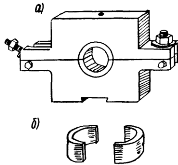
Рис. 23. Охладитель со сменными вкладышами: a - охладитель; b - сменные вкладыши
