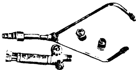
Рис. 21. Двухрожковая пропано-кислородная горелка
