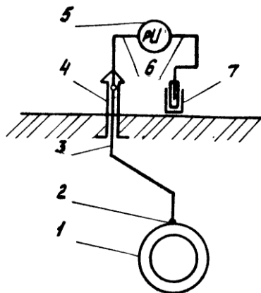
Рис. 31. Схема измерений разности потенциалов «труба-земля»:
