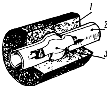
Рис. 9. Термитный патрон марки АС для сварки жил проводов и кабелей: 1 - термитный патрон; 2 - кокиль; 3 - алюминиевый вкладыш
