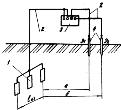
Рис. 30. Схема измерения сопротивления растеканию тока анодного заземления:
