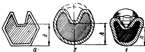
Рис. 28. Измерение остаточной толщины в месте опрессовки:
