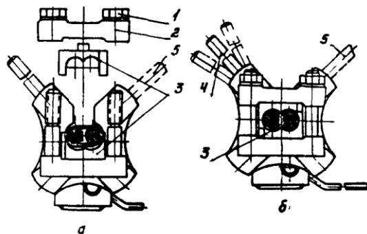
Рис.7. Зажимные узлы приспособления МИ-230А:
