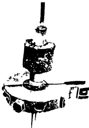
Рис.18. Введение стального стержня в кокиль термитного патрона с расплавленным алюминием
