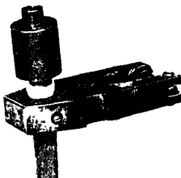
Рис.16. Патрон марки АС с охладителем, установленный для сварки алюминиевой жилы кабеля со стальным стержнем
