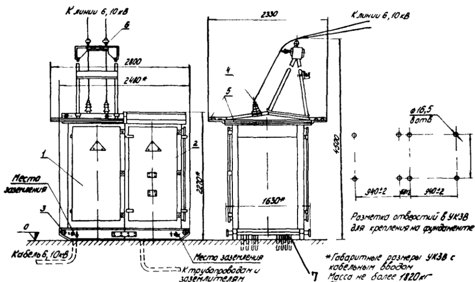
Рис. 2. Общий вид смонтированного устройства катодной защиты высоковольтного УКЗВ: 1 - блок высоковольтного трансформатора; 2 - блок катодных станций; 3 - салазки; 4 - изолятор проходной; 5 - сетка ограждения; 6 - кронштейн воздушного ввода; 7 - труба кабельного ввода
