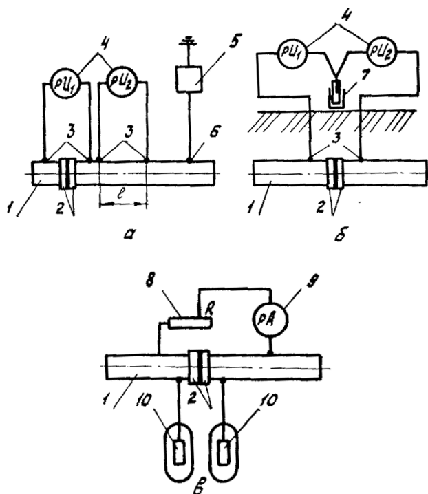
Рис. 34. Схемы включения измерительных приборов и устройств при опробовании и наладке изолирующих фланцев трубопровода:
