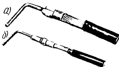
Рис.19. Образцы контактных соединений стальных стержней с алюминиевыми жилами кабеля: а - с разрезом сварного соединения; б - без разреза сварного соединения
