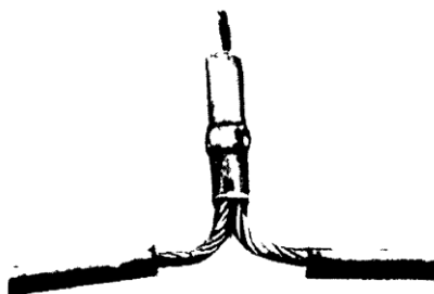
Рис.14. Образец контактного соединения проводов марки ПСРП с алюминиевыми жилами кабеля
